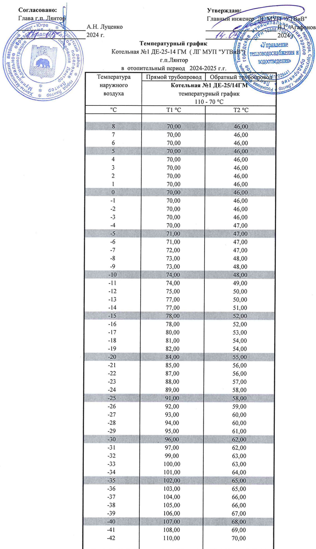
Рисунок 4. Температурный график регулирования отпуска тепловой энергии от котельной №1
