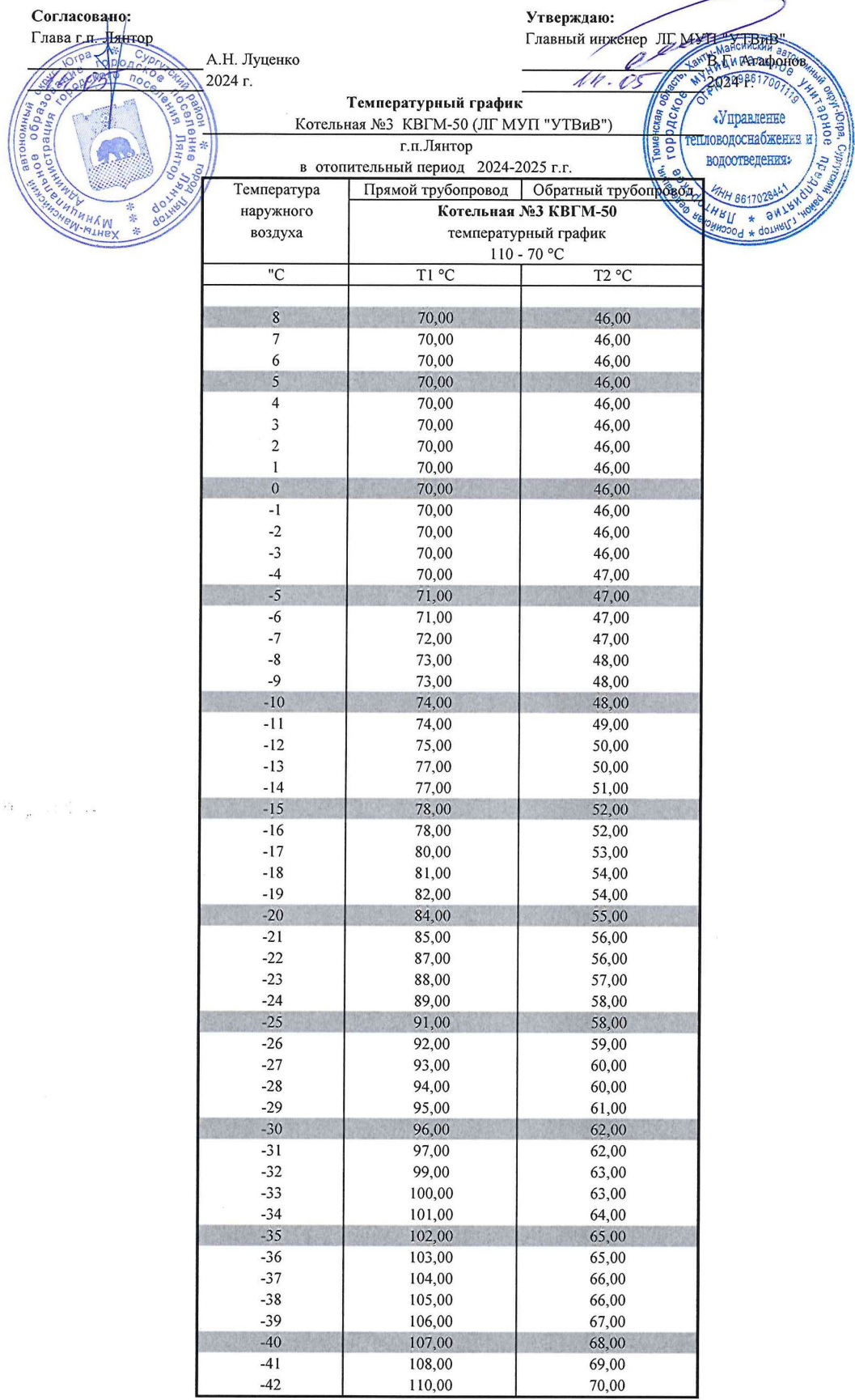
Рисунок 6. Температурный график регулирования отпуска тепловой энергии от котельной №3
